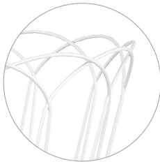
Tondino di acciaio zincato piegato con macchine a controllo numerico, per una maggiore precisione ed un migliore controllo del processo produttivo. Hot-dip zinced steel bar bent with numerical control machines for a more precise and accurate manufacturing process.
